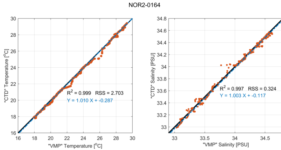
圖 4、紊流儀 VMP-250 SN474 之(a)溫度與(b)鹽度資料和新海研 2 號 CTD 資料比較。
