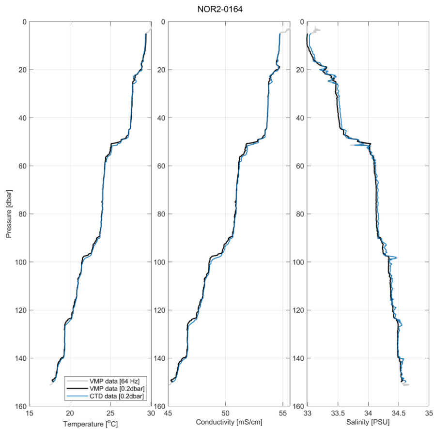
圖 3、紊流儀 VMP-250 SN474 之(a)溫度、(b)導電度與(c)鹽度資料與新海研 2 號 CTD 資料比較。
