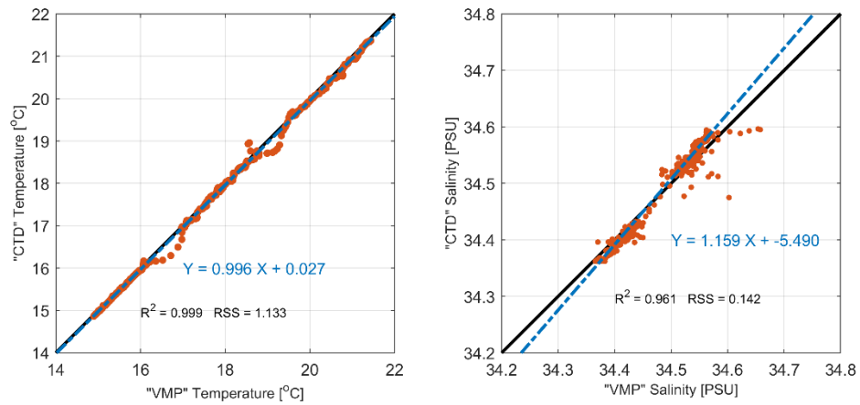
圖 2、紊流儀 VMP-250 SN474 之(a)溫度與(b)鹽度資料和新海研 2 號 CTD 資料比較。
