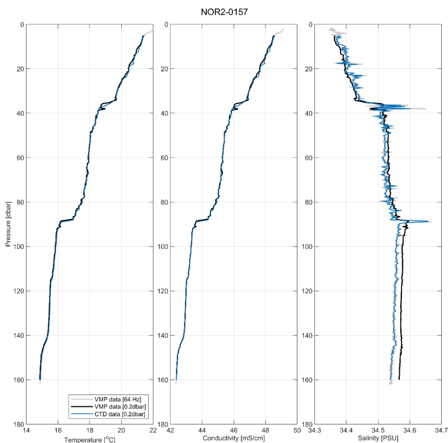
圖 1、紊流儀 VMP-250 SN474 之(a)溫度、(b)導電度與(c)鹽度資料與新海研 2 號 CTD 資料比較
