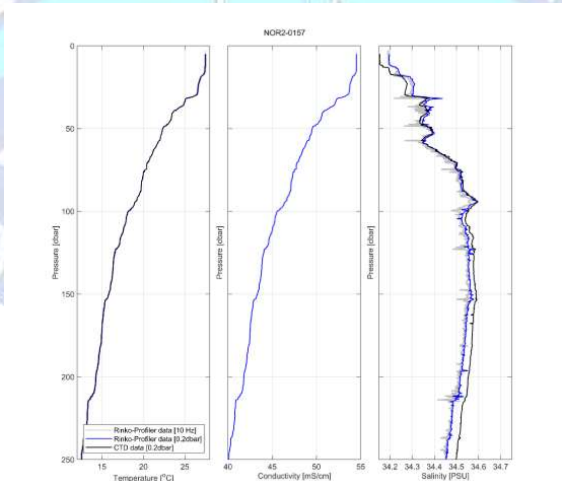
圖 1、RINKO-Profiler SN844(a)溫度、(b)導電度與(c)鹽度資料與新海研 2 號 CTD 資料比較
