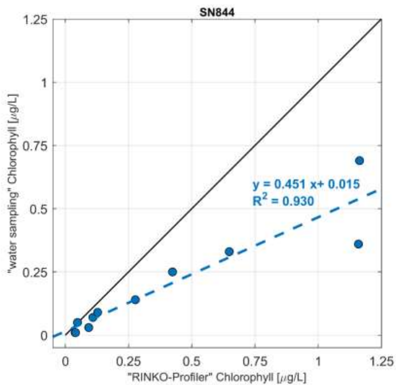
圖 3、RINKO-Profiler SN844 葉綠素 a 資料與海水採樣資料相比較。
